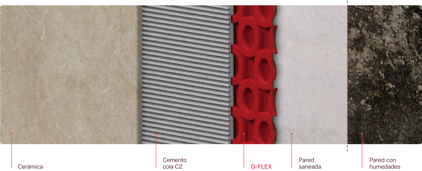
Humedad negativa con acabado cerámico
