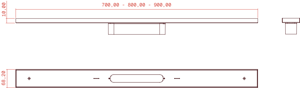
Canaletta lineare antivandalo
