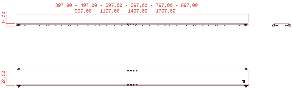
Griglia Lisa lineare
