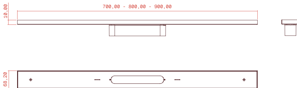
Canaleta Lineal Antivandal.
