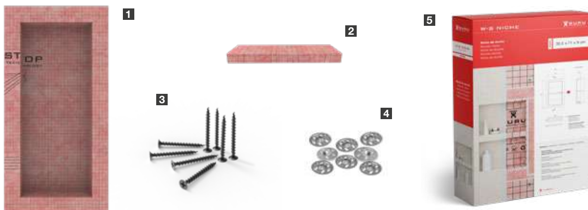
1- Nicchia prefabbricata W-S NICHE. 2- Ripiano. 3- Viti (x8). 4- Rondelle metalliche (x8). 5- Scatola W-S NICHE.
