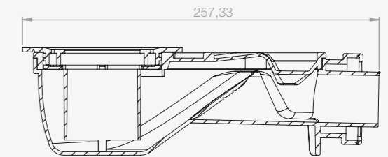
SECCIÓN B-B
