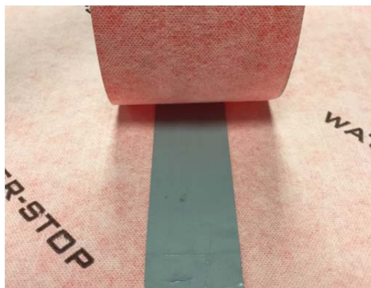
Figura.- Realización de la unión del solape con masilla W-S MASTIC
